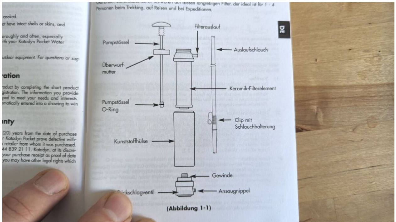
Der Aufbau vom Katadyn Pocket Wasserfilter
